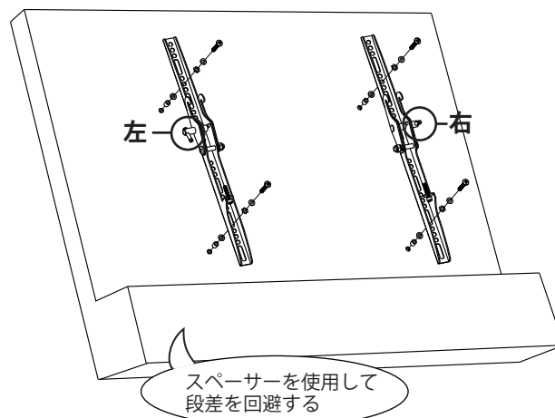
取付け順序 M4/M5 ボルト取付けの場合
